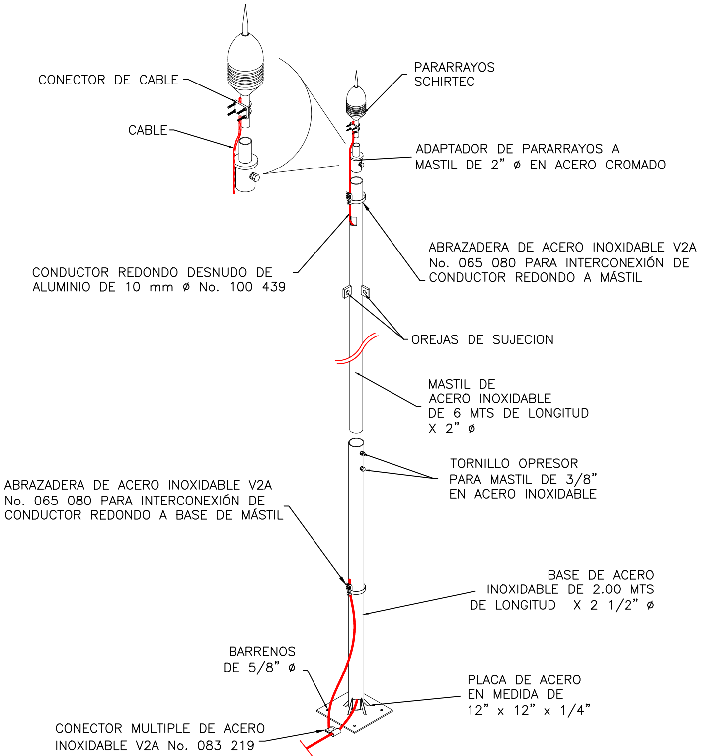
DETALLE DEL SOPORTE DE PUNTA PARARRAYOS SCHIRTEC SIN ESCALA.
